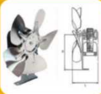
Ventilatore assiale bassa portata
