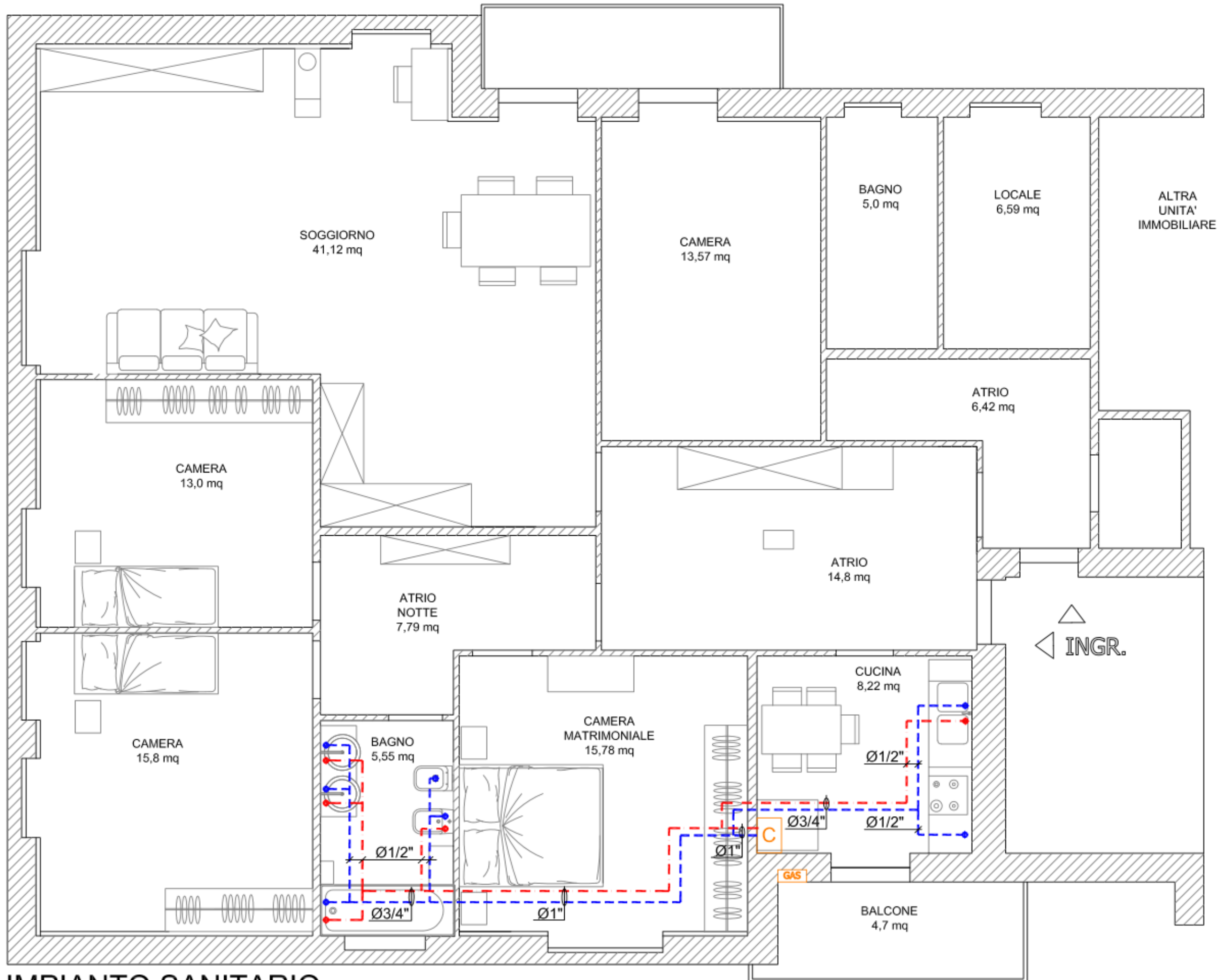
IMPIANTO SANITARIO
