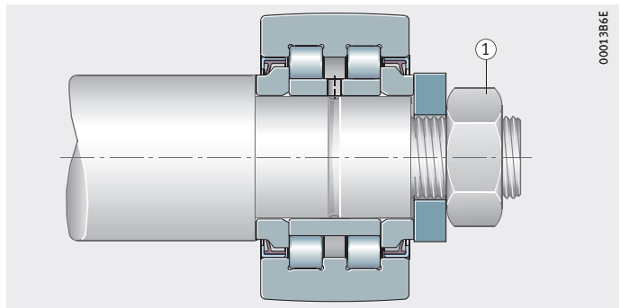
Figura 21 Bloccaggio assiale
