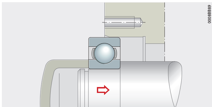
Figura 1 Montaggio di un cuscinetto non scomponibile
