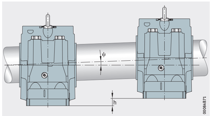
Figura 8 Disassamento dell'albero
