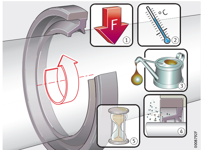
Figura 1 Fattori di influenza della durata d'esercizio delle tenute
