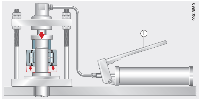
Figura 20 Montare il rullo di appoggio con pressa di montaggio
