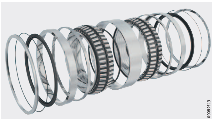
Figura 11 Cuscinetti a rulli conici a quattro corone
