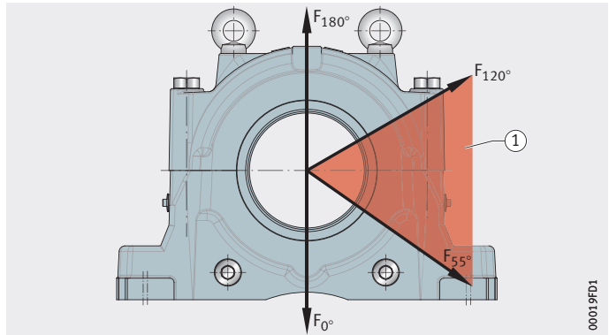
Figura 9 Direzioni di carico in un supporto ritto
