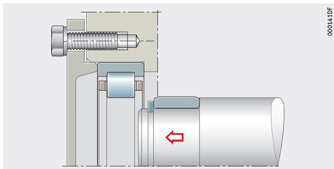
Figura 2 Montaggio di un cuscinetto scomponibile
