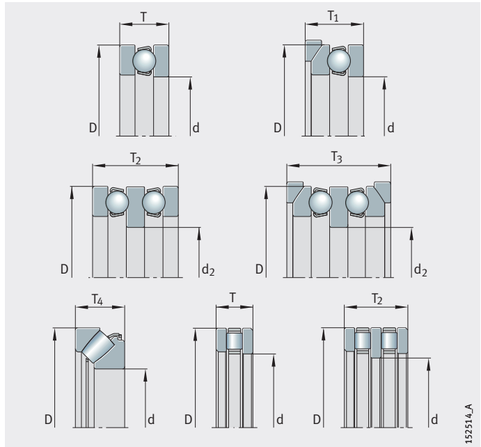
Figura 1 Tolleranze dell'altezza nominale del cuscinetto
