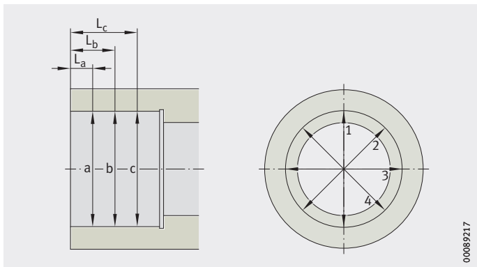
Figura 2 Alloggiamento
