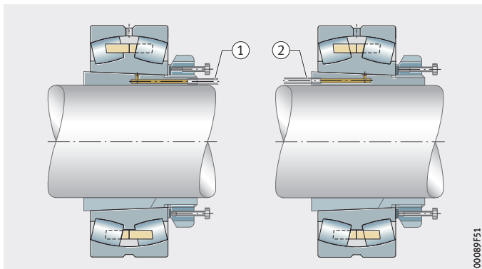
Figura 26 Sede del cuscinetto sulla bussola di trazione
