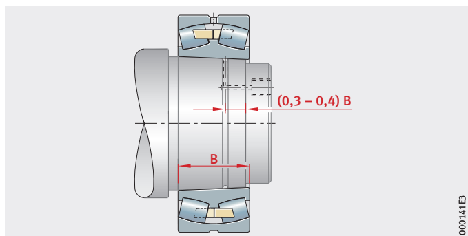
Figura 23 Larghezza consigliata per gole dell'olio
