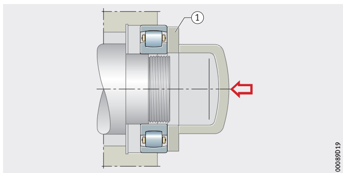
Figura 5 Calettamento contemporaneo con disco di montaggio
